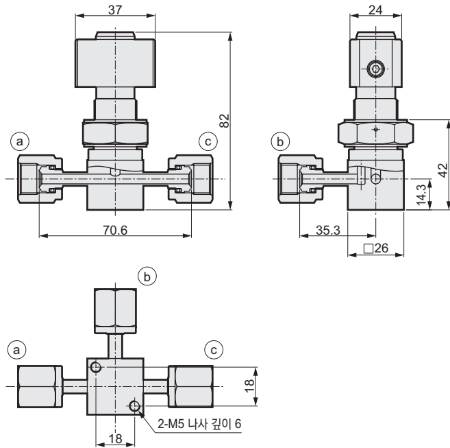
그림은 OGD10R-4RJ-FFF-K 암피팅(베어링 포함)
