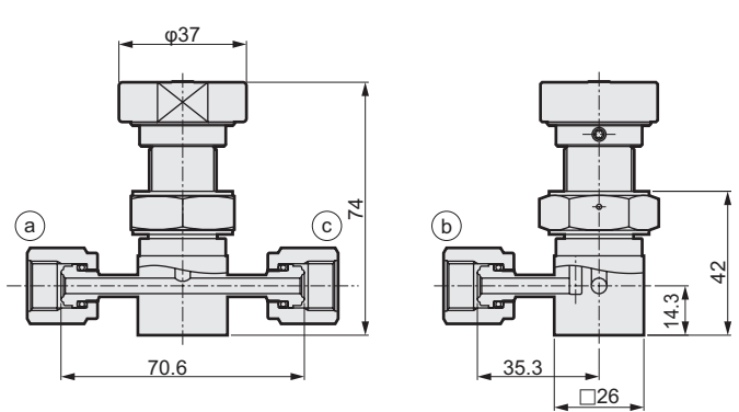
그림은 MGD10R-4RJ-FFF-K 암피팅(베어링 포함)
