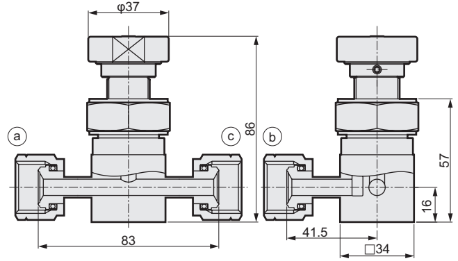
그림은 MGD20R-6RJ-FFF 암피팅(베어링 포함)
