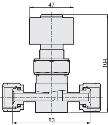
그림은 OGD20R-6RJ-K 암피팅(베어링 포함)
